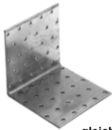
gleichschenkelig
