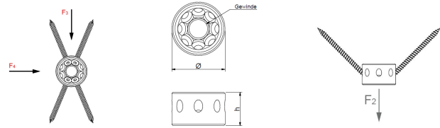
Schraubenbild 4
