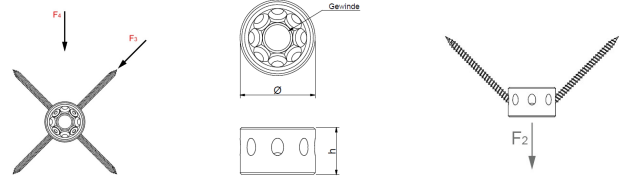
Schraubenbild 2
