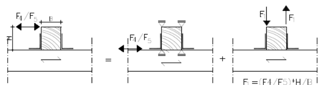
Abb. 3: Lastfall F_4/F_5 zurückgeführt auf zwei Grundlastfälle
