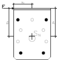
Abb. 6: Horizontaler Schenkel, Abscherbeanspruchung
