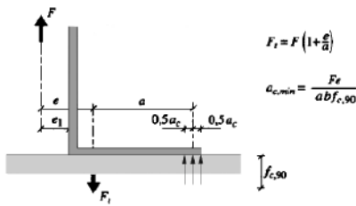
Abb. 4: Statisches Modell Lastfall F_1
