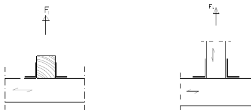
Abb. 1: Belastung durch F_1 , Schwelle und Stütze
