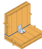
Winkelverbinder befestigt mit SDS Schraube
