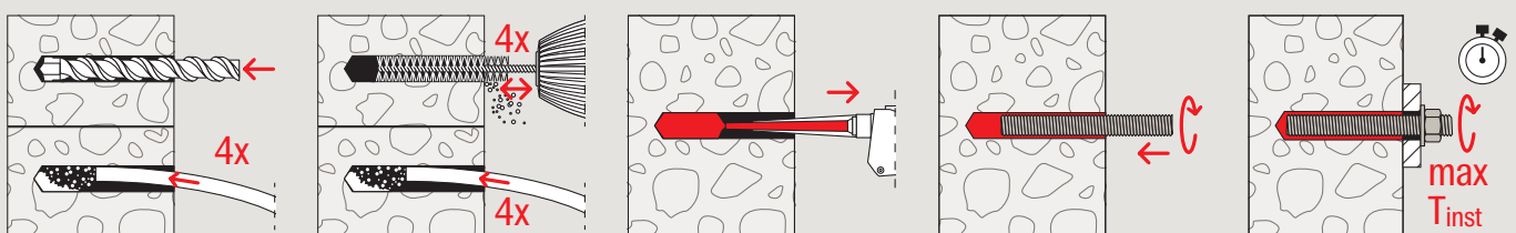
Montage exemplarisch für Ankerstange FIS A in Beton
