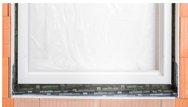
10. Fertig Fertiger luftdichter bzw. schlagregensicherer Anschluss. Band kann jetzt überputzt werden.
