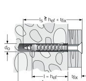
Dübel SX mit Schraube
