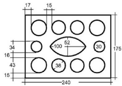
Bild 4 KSL 12-1.4 - 3DF
