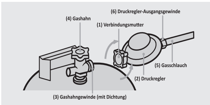
Abb.2: Montage des Druckreglers
