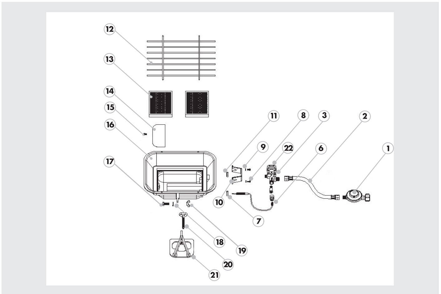
Abb. 4: Explosionszeichnung
